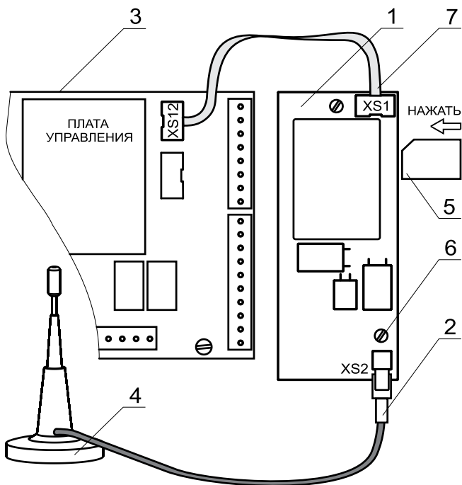
Рис.1 Подключение модуля GSM к пеллетному котлу Zota Pellet
