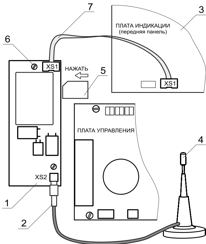
Рис.1 Подключение модуля GSM к угольному котлу Zota Стаханов
